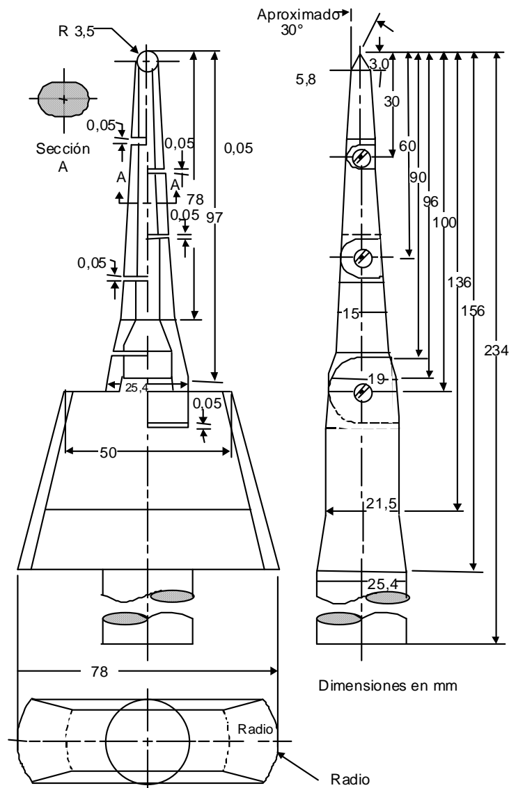
Figura 2.- Sonda de prueba articulada
