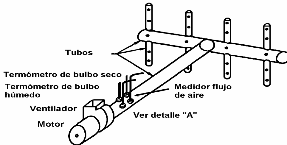
Figura C.1 Dispositivo de toma de muestra de aire para la unidad de prueba o el equipo de acondicionamiento.
